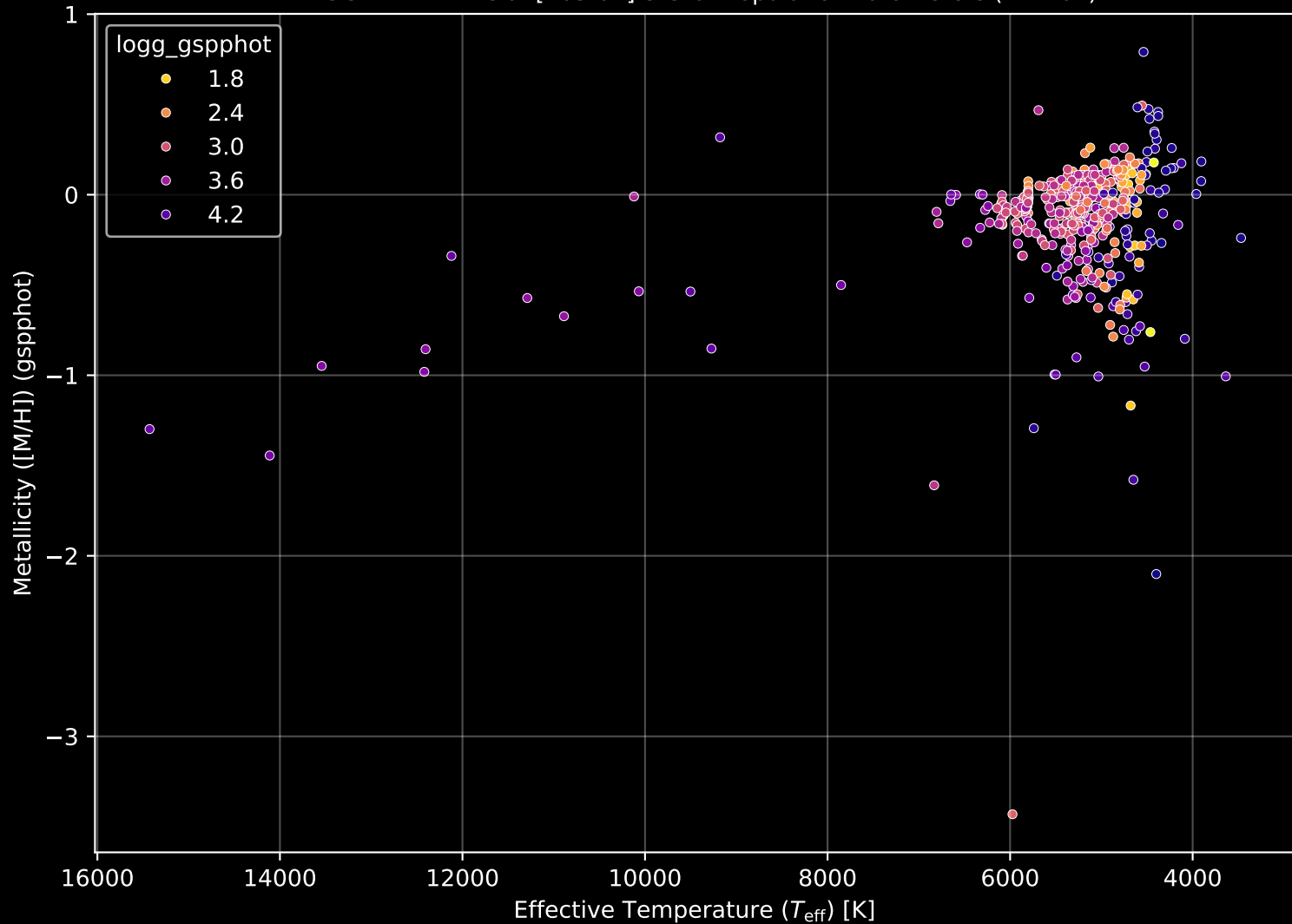
APOGEE DR17 Field: [165-04] Stellar Population Parameters (n= 461)
